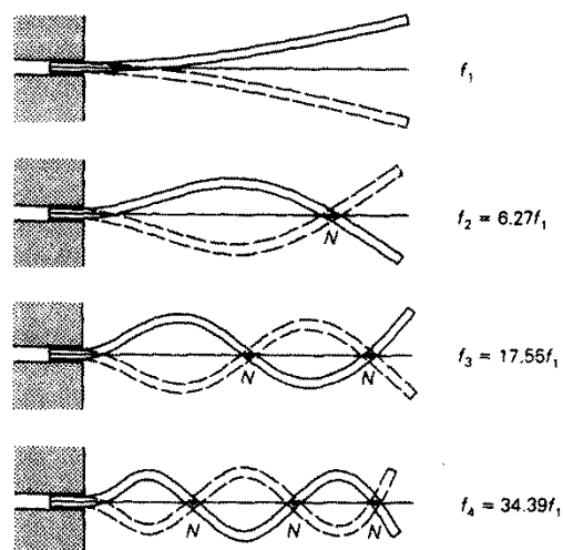
Knopen en buiken in een trillende plaat, die aan één zijde is vastgeklemd. Naar Rossing.
