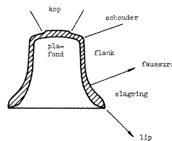
Profiel van een klok Naar Lehr 1976, p. 4
