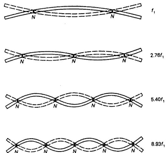
Knopen en buiken in een plaat met vrije uiteinden aan beide zijden. Naar Rossing.
